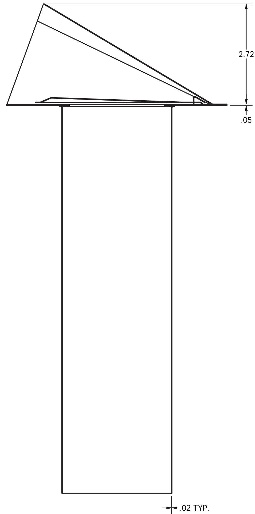
SECTION A-A
